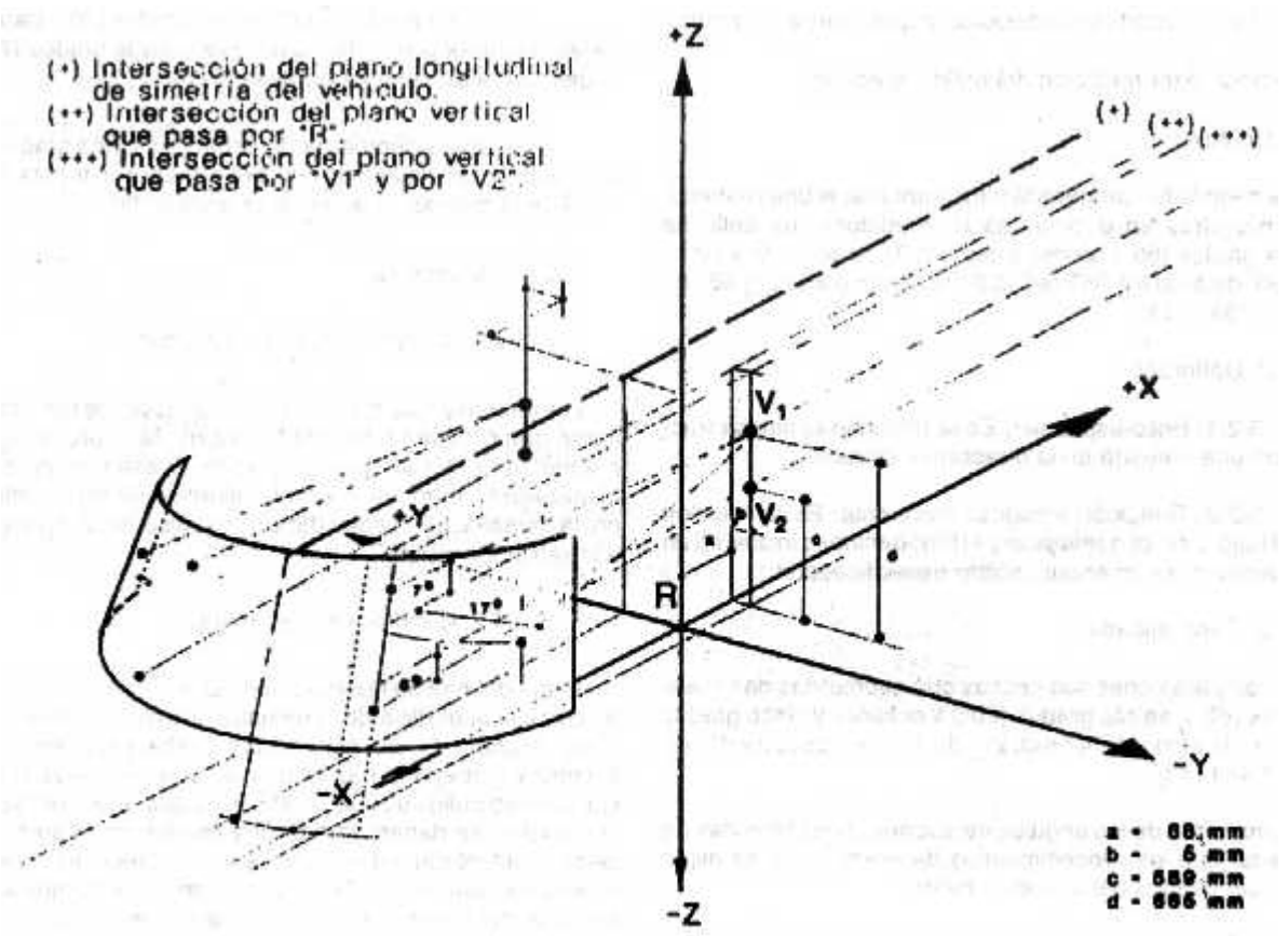
Figura 20 - Determinación de puntos V para un ángulo de incidencia de 25°.
