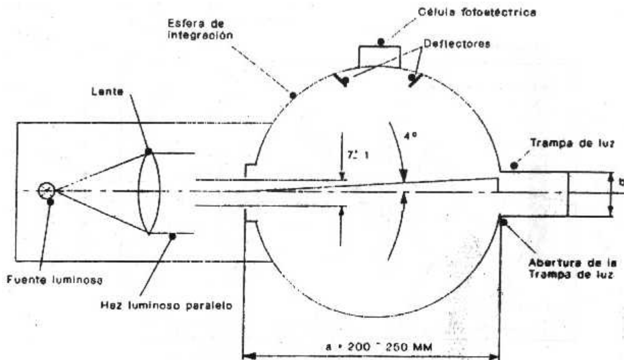
Figura 5 - Medidor de Atenuación de visibilidad
