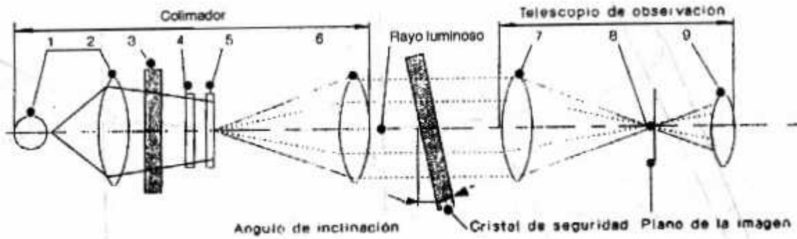
Figura 13 · Aparato para el ensayo con el colimador
