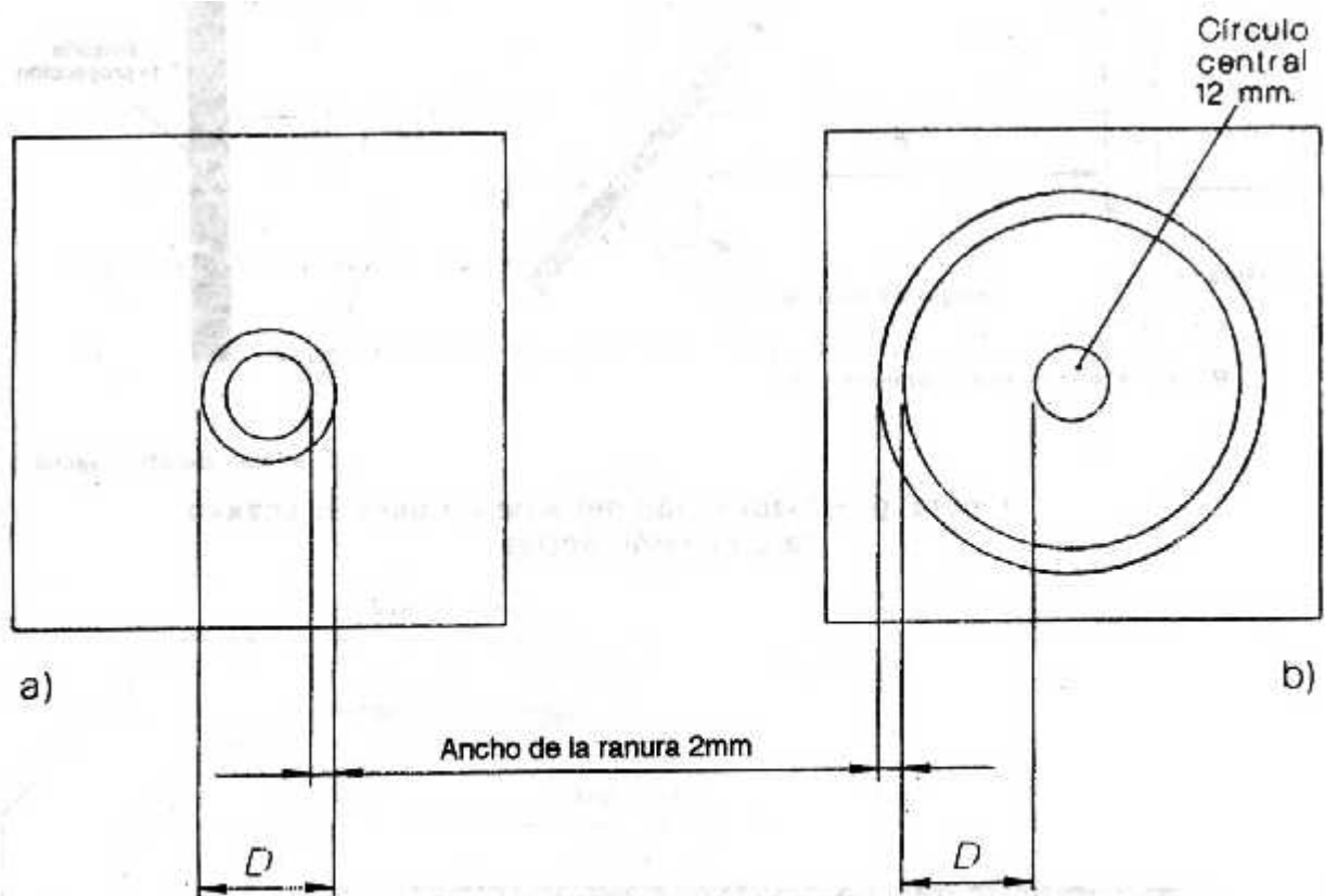
Figura 11 - Dimensiones del objetivo
