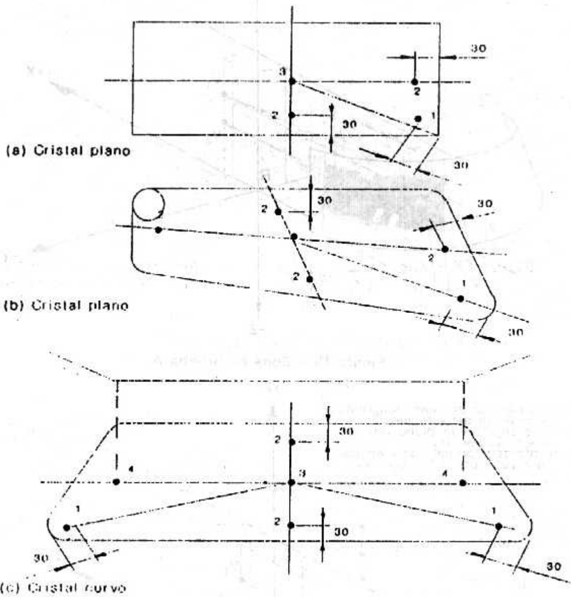
Figura 17 (a), 17 (b) y 17 (c) - Puntos de impacto prescritos para cristales laterales y lunetas
