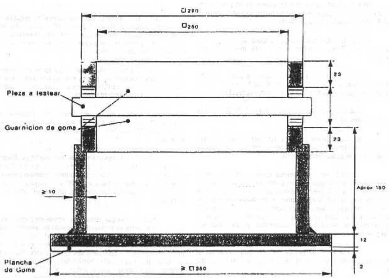
Figura 1 - Soporte para ensayo de caída de bola.
