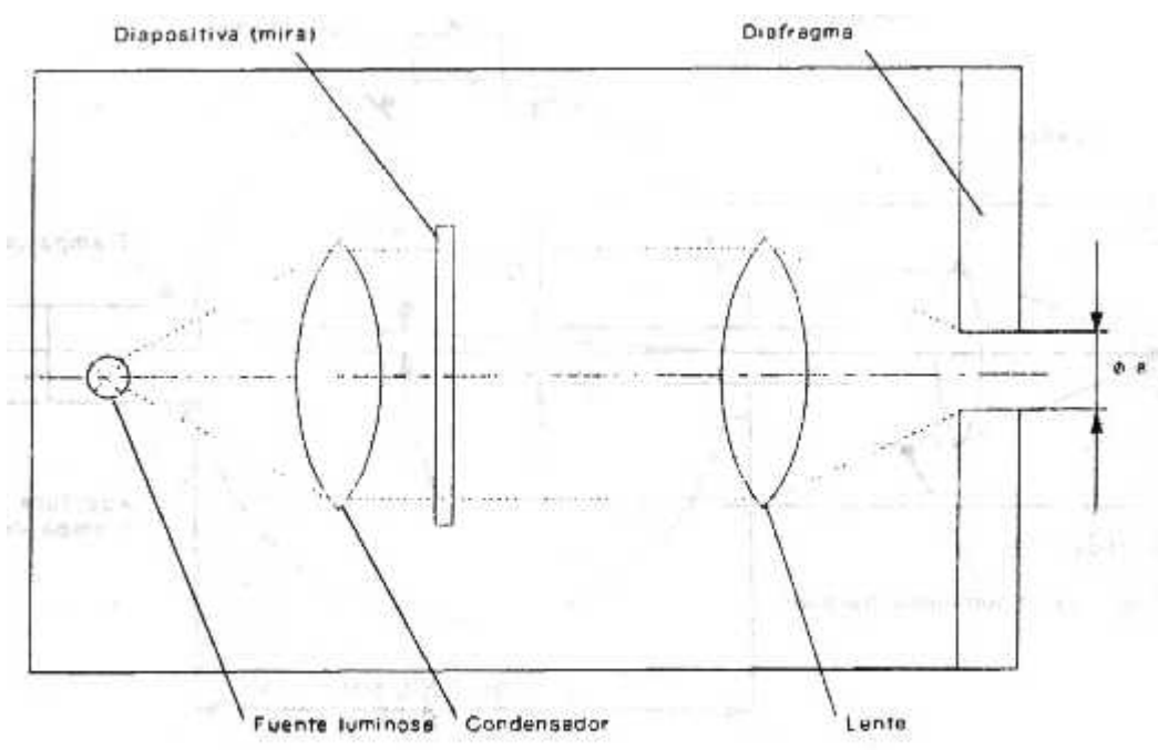
Figura 7 - Esquema óptico del proyector
