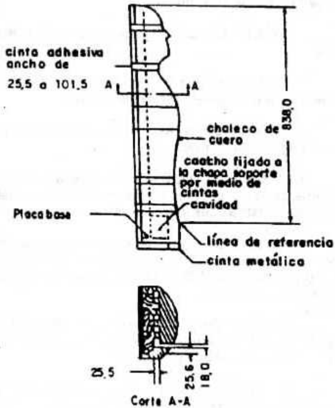
FIG. 4-PERFIL DEL BLOQUE
