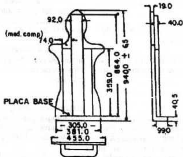
FIG. 3 - CHAPA SOPORTE
