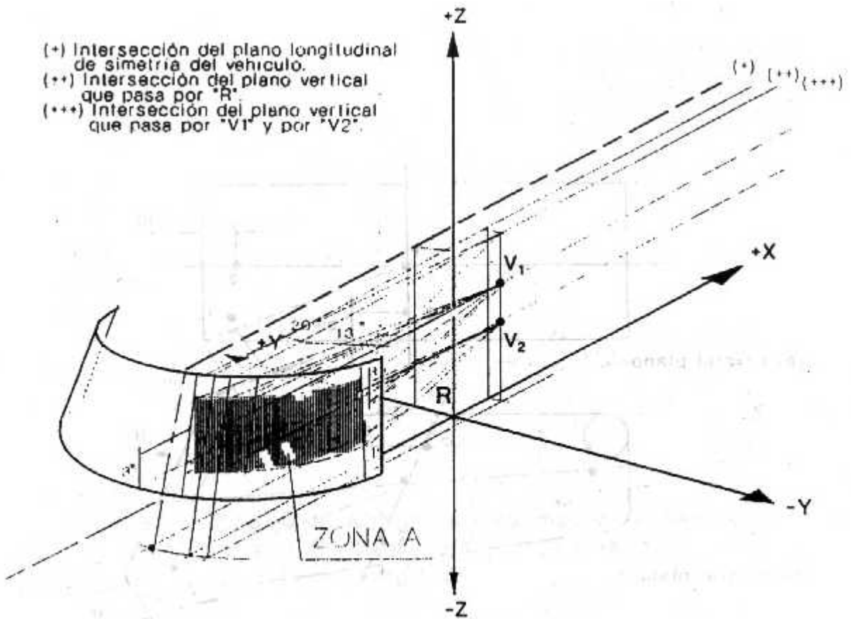
Figura 18 - Zona de prueba A
