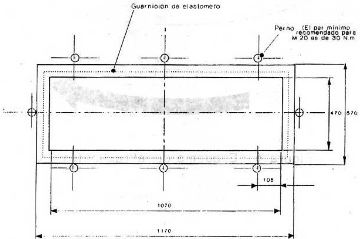
Figura 3 - Soporte de cabeza de prueba
