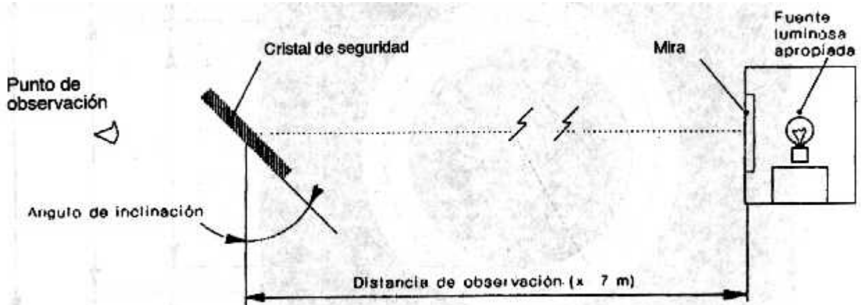
Figura 12 - Disposición del aparato.
