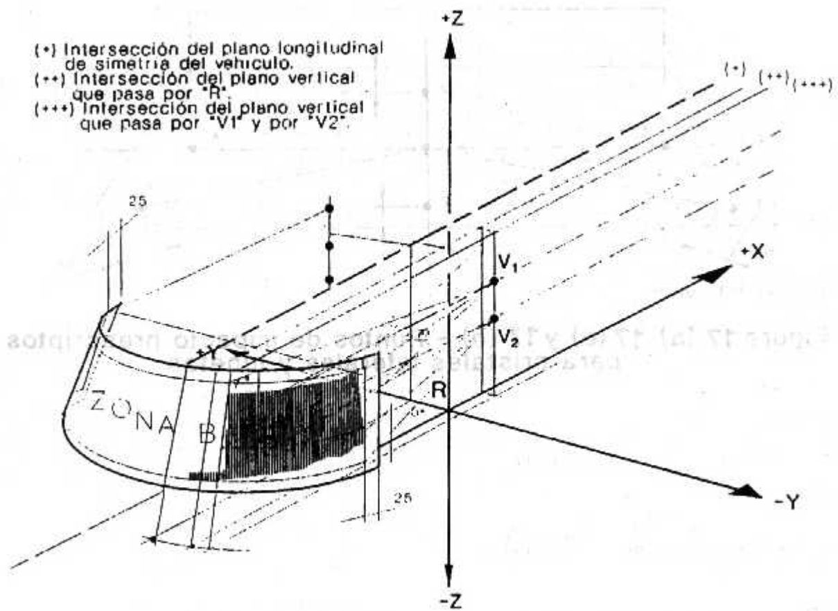
Figura 19 - Zona de prueba B
