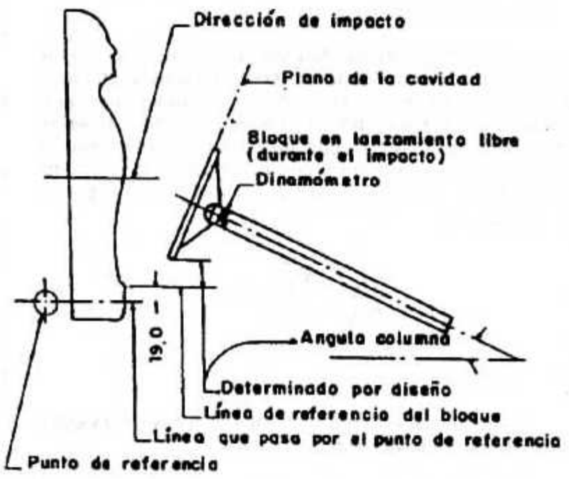
FIG. 5 - RELACION ENTRE EL SISTEMA DE DIRECCION Y DEL BLOQUE.
