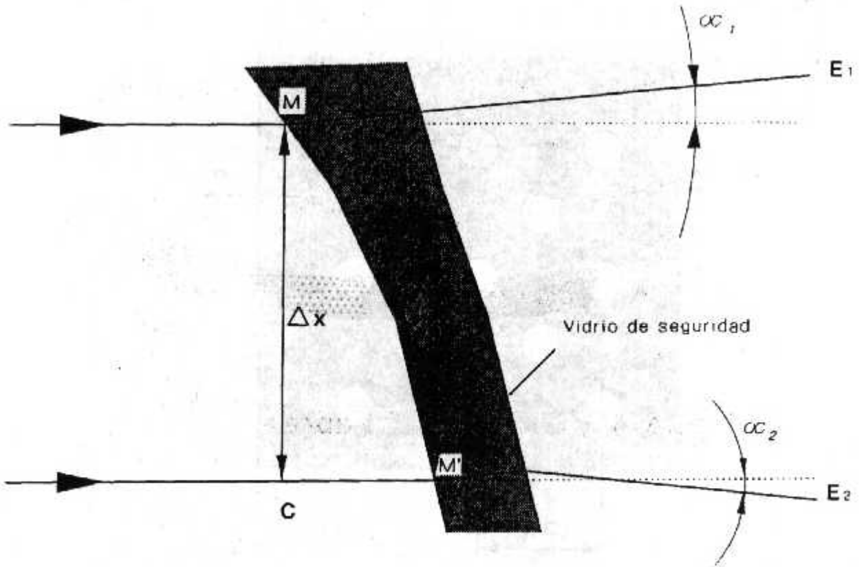
Figura 6 - Representación esquemática de la distorsión óptica.
