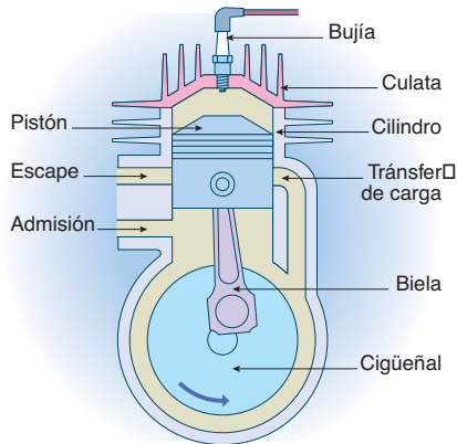
Esquema de un motor de 2 tiempos
