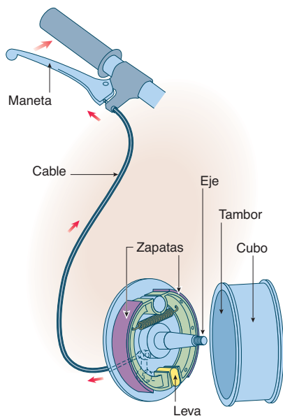
Funcionamiento de un freno de tambor
