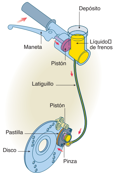
Funcionamiento de un freno de disco
