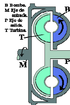
Fig. 7-11 Embrague hidráulico
