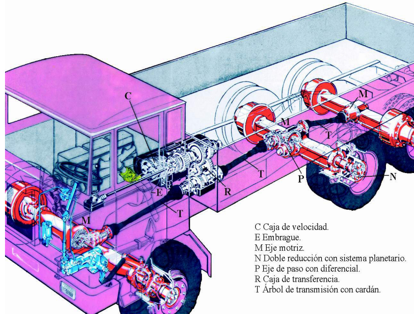
Fig. 1-1 Organización del automóvil
