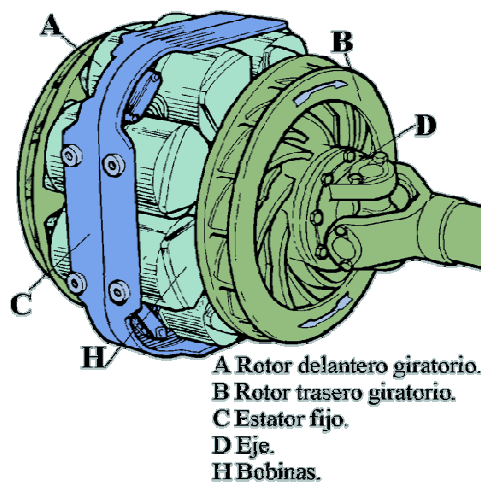
Fig. 10-14 Freno eléctrico
