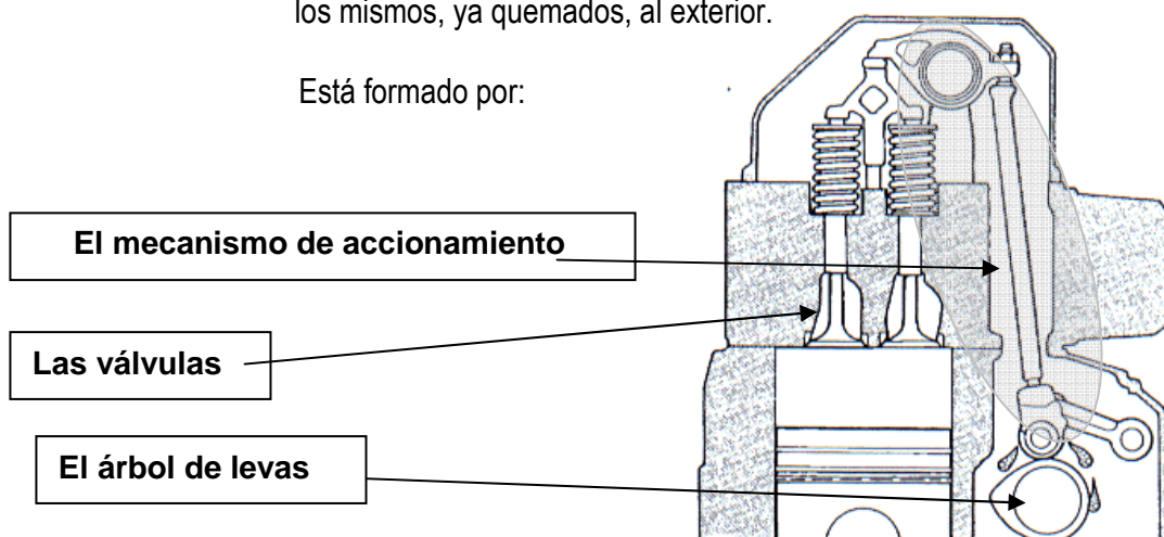
Fig. 2-10 Sistema de Distribución
