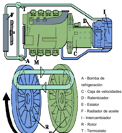
Fig. 10-11 Ralentizador
