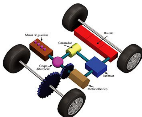
Fig. 2-1 Motor híbrido
