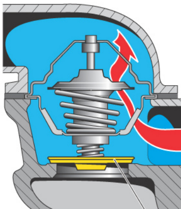
Fig. 5-20 Termostato abierto
