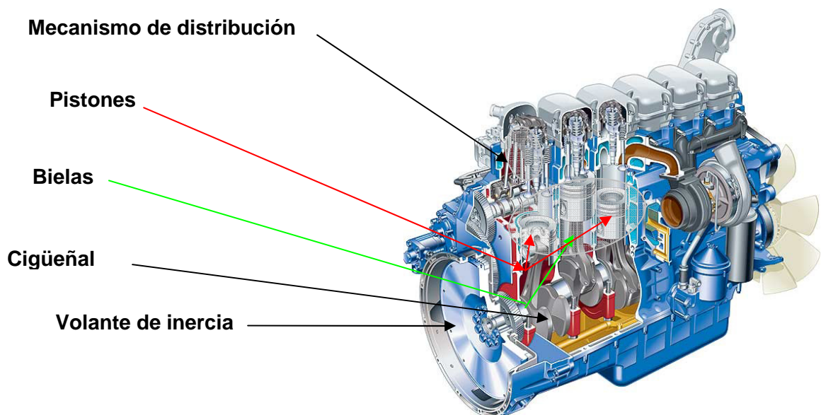
Fig. 2-3 Elementos móviles
