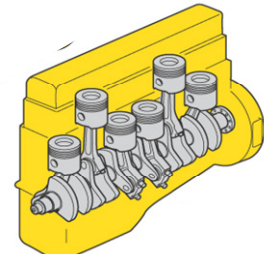
Fig. 2-13 Motor de 6 cilindros en línea
