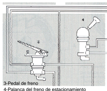
Fig. 10-8 Elementos de mando
