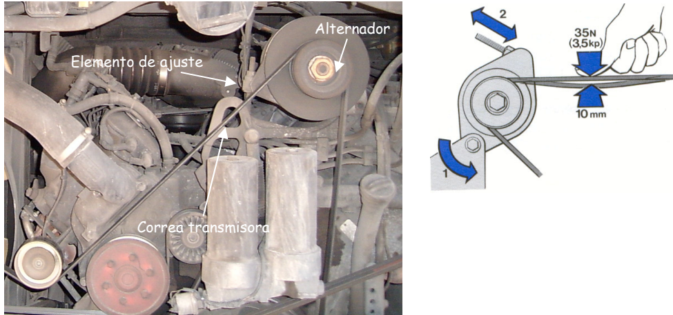
Fig. 6-9 Situación del alternador y ajuste de la correa
