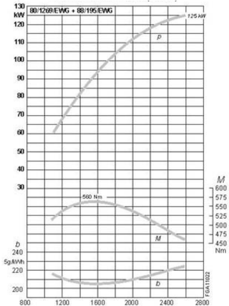
Fig. 2-23 Curvas de par, potencia y consumo
