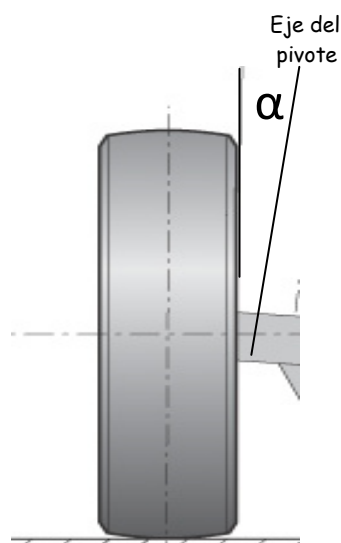
Fig. 9-9 Ángulo de salida
