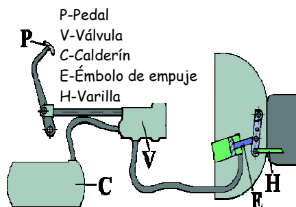
Fig. 7-10 Accionamiento neumático
