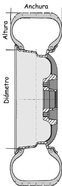
Fig. 8-12 Cotas dimensionales
