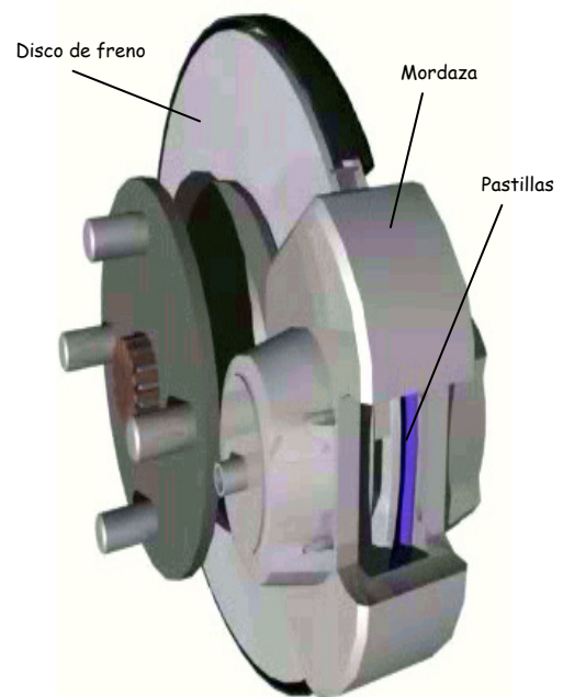
Fig. 10-3 Freno de disco
