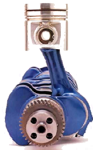
Fig. 2-8 Unión Pistón-Biela-Cigüeñal
