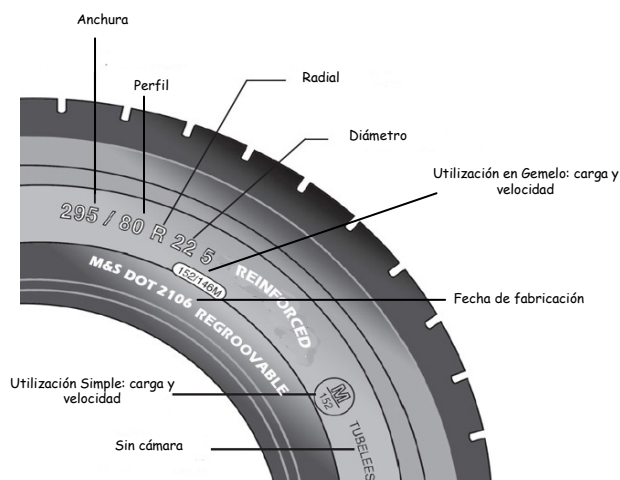
Fig. 8-13 Marcado del neumático, en el flanco
