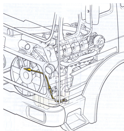
Fig. 5-12 Varilla de control del nivel de aceite
