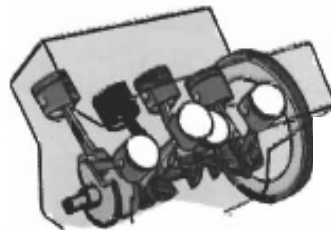
Fig. 2-14 Motor de 8 cilindros en V
