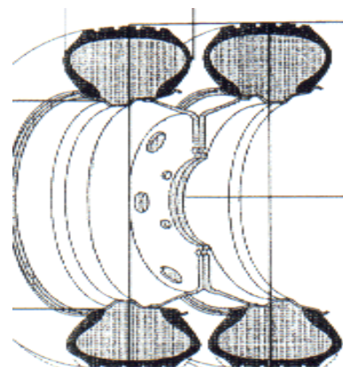
Fig. 8-14 Montaje gemelo
