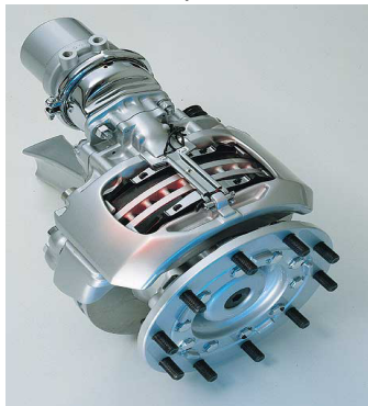
Fig. 10-4 Discos ventilados
