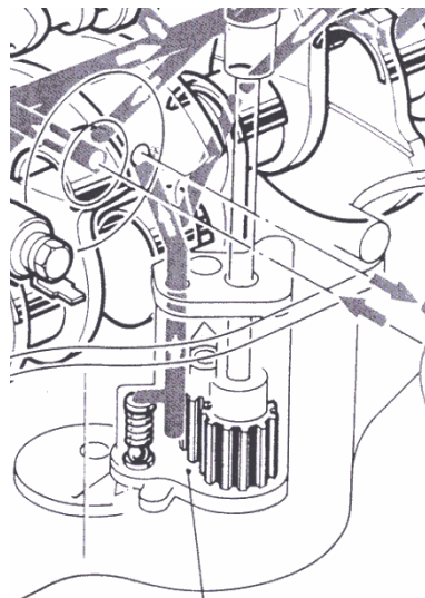
Fig. 5-4 Bomba de aceite
