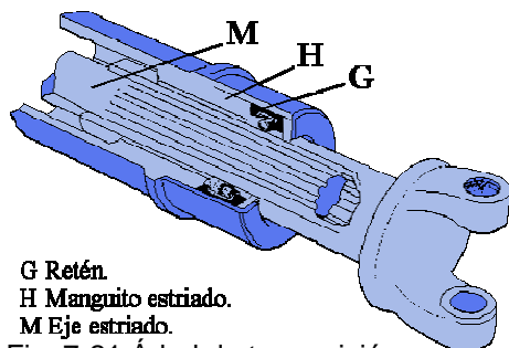
Fig. 7-21 Árbol de transmisión extensible
