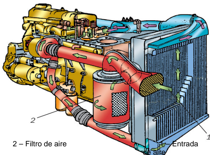
Fig. 3-1 Sistema de alimentación
