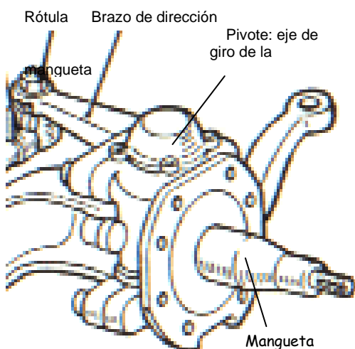
Fig. 9-5 Conjunto de mangueta-pivote
