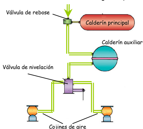
Fig. 9-18 Instalación básica del sistema neumático
