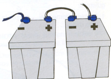
Fig. 6-6 Conexión serie
