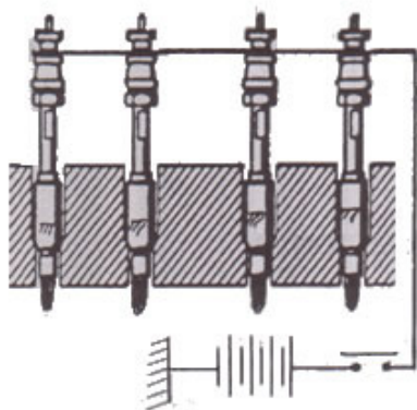
Fig. 3-8 Conexión en paralelo
