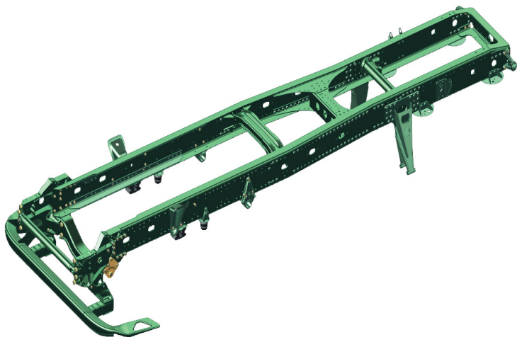
Fig. 1-3 Bastidor convencional
