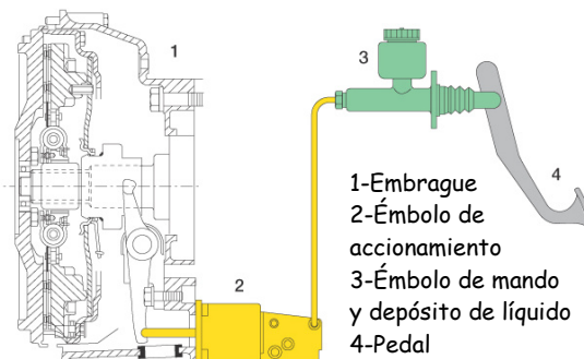
Fig. 7-9 Accionamiento hidráulico
