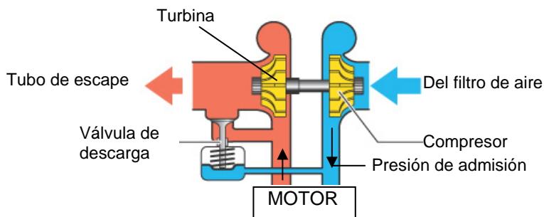
Fig. 3-10 Montaje de la válvula de descarga
