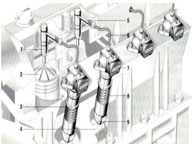
Fig. 3-16 Sistema bomba-inyector
