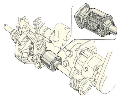
Fig. 7-27 Bloqueo del diferencial
