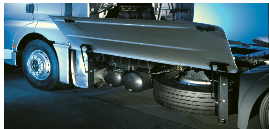
Fig. 1-8 Colocación depósitos de aire comprimido y rueda de repuesto
